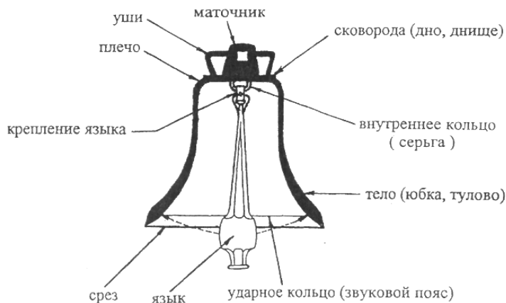
Рис. 4. Примерный вид колокола и его основные части
